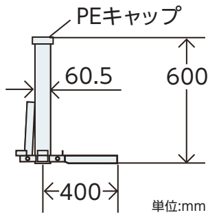
横面図
